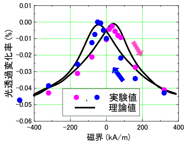
図2. (a) 660°Cに加熱したガラス基板(コーニング社製イーグル2000)上に作製した \text{Fe}_9\text{Co}_5\text{Al}_{19}\text{F}_{67} ナノグラニューラー膜(1 \mu\text{m} )の写真。膜は透明で、後ろの赤、青、黄色の文字をくっきりと見ることができます。(b) \text{Fe}_{13}\text{Co}_{10}\text{Al}_{22}\text{F}_{55} ナノグラニューラー膜の光透過率の変化(波長: 1500nm)。丸印は実験値で実線は理論値です。これは、スピン依存電荷振動による『トンネル磁気誘電効果』に基づく、従来に無い新しい磁気-光学効果です。
